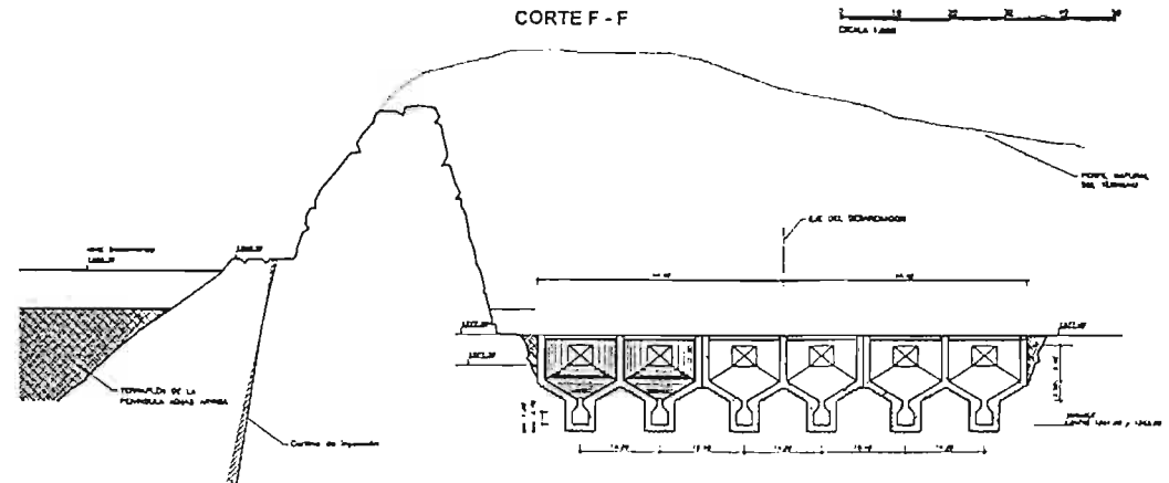
CORTE LONGITUDINAL DEL SIFON CORTE B-B
