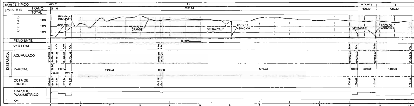
TUNEL DE CONDUCCIÓN TRAMO: CAPTACIÓN - VENTANA 2 ( 10883.32 m)
