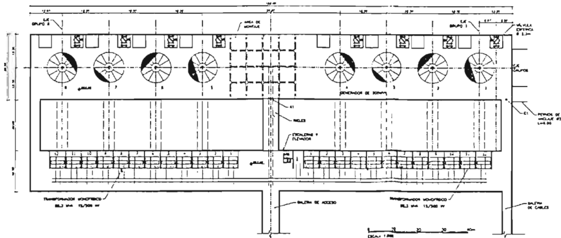
PISO PRINCIPAL Y DE TRANSFORMADORES
