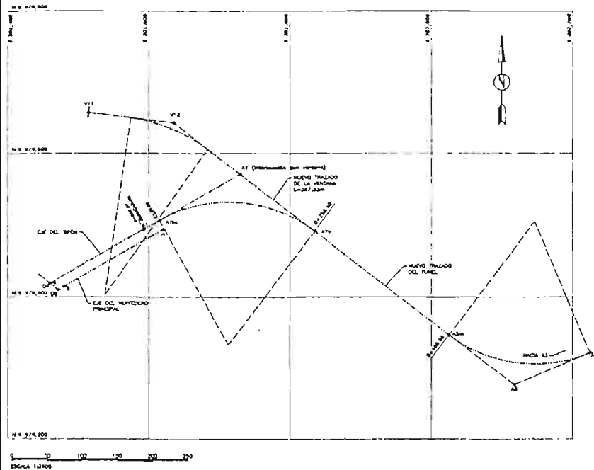
TRAZADO VENTANA 1 EMBOCADURA TUNEL
