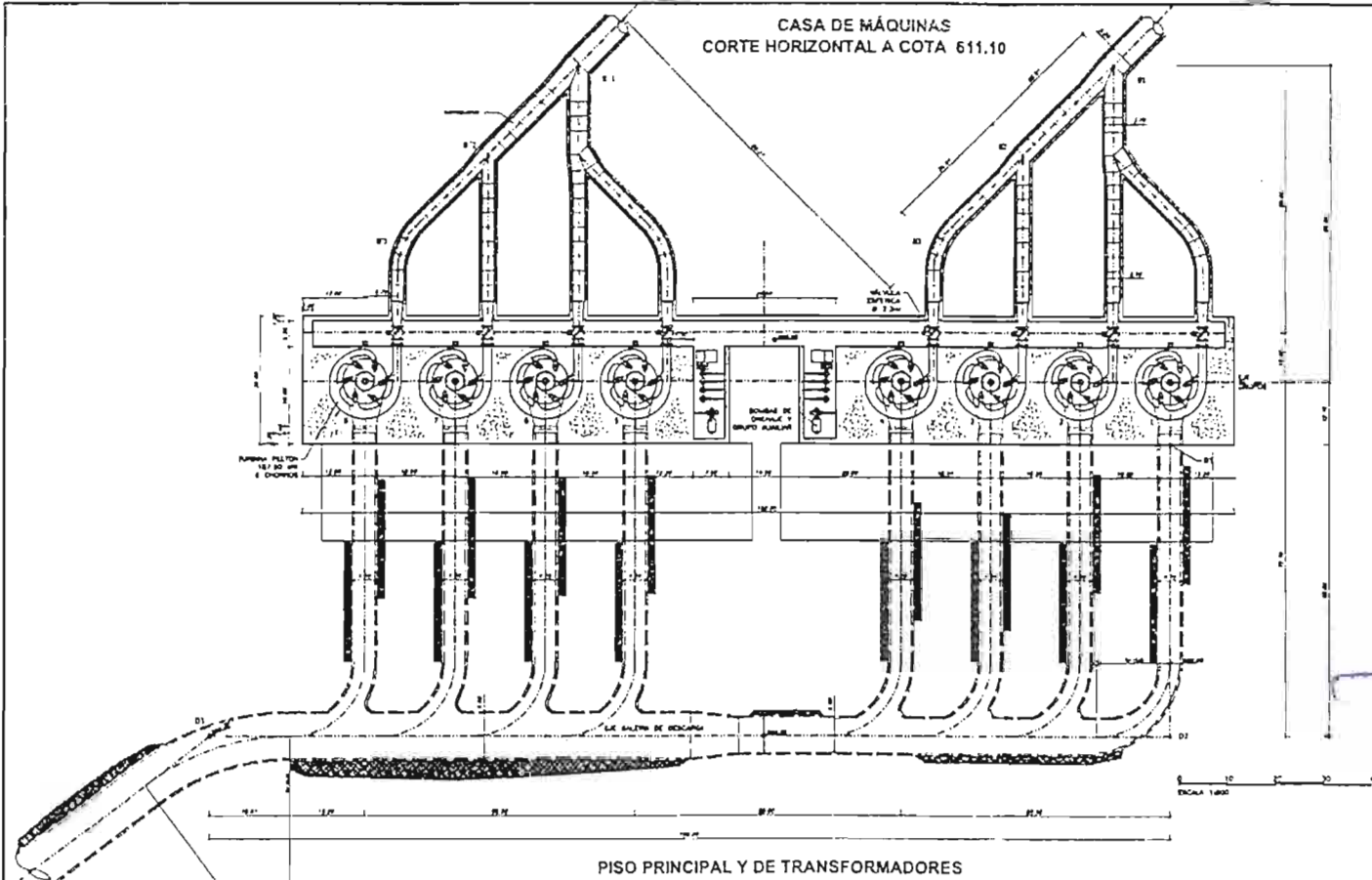
PISO PRINCIPAL Y DE TRANSFORMADORES
