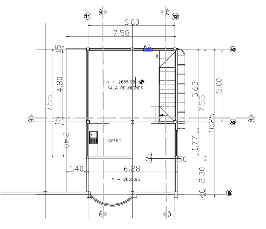
P.A.2 OFICINAS ESC. 1:100 N° 2655.95
