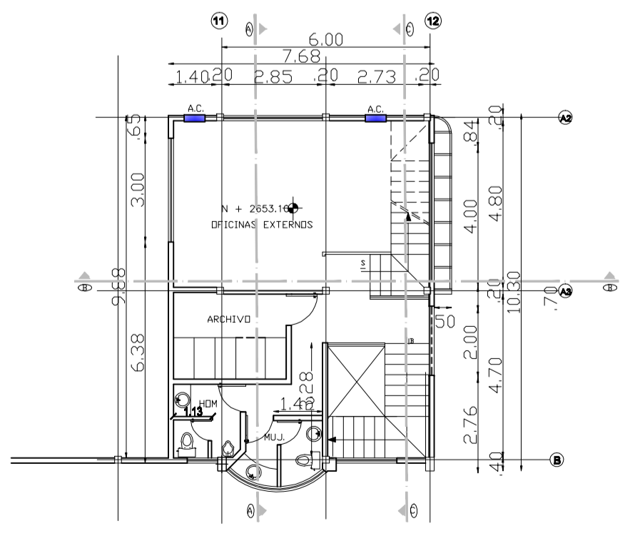
P.A.1 OFICINAS ESC. 1:100 N° 2653.19
